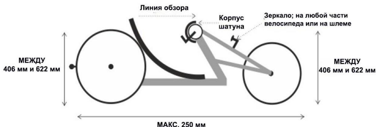
Рисунок 8. Ручной велосипед, приводимый в движение силой рук, в лежачем положении.
