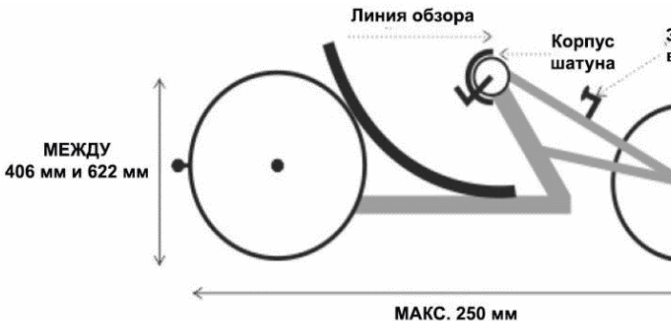
Рисунок 8. Ручной велосипед, приводимый в движение силой рук, в лежачем положении.
